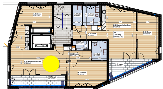
Grundriss 1. OG Haus 2 „Linde“
